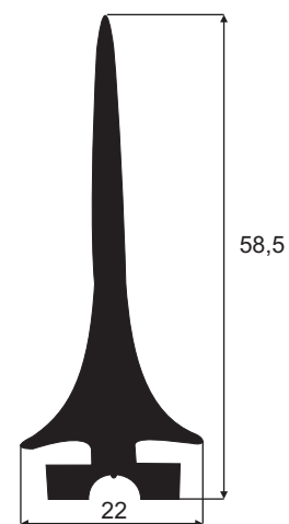
IBC 3383 EPDM 80 Sh A
