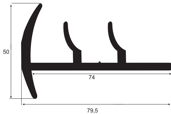
IBC 3413 EPDM 75 Sh A Vedação Porta Frigorífico
