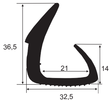
IBC 3277 SBR 80 Sh A Vedação Porta Container
