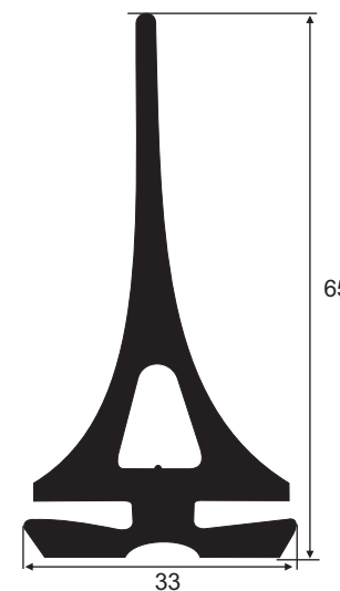
IBC 3445 EPDM 70 Sh A
