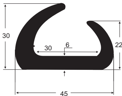
IBC 3564 EPDM 75 Sh A
