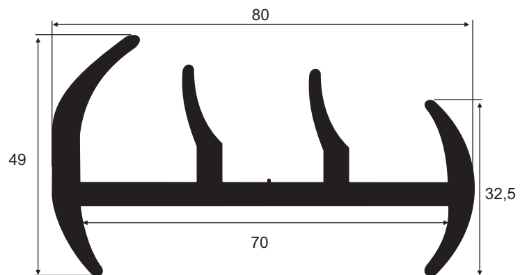
IBC 3379 EPDM 70 Sh A Vedação Furgões Frigoríficos Randon
