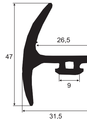
IBC 3445 EPDM 70 Sh A
